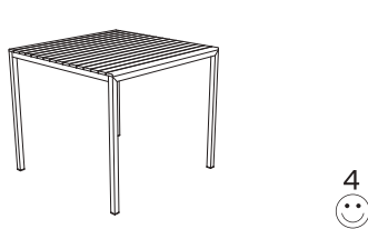
LCR615 86,5 × 86,5 × 76,5 cm
