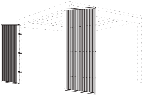
SOP300 270 × 259,5 cm
