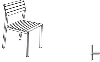
LCR126 49,5 × 58 × 85 cm
